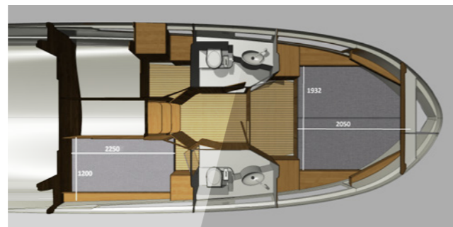
Wersja 2 kabinowa, koja dziobowa i rufowa / EN / 2-cabin layout, forward and aft cabin
