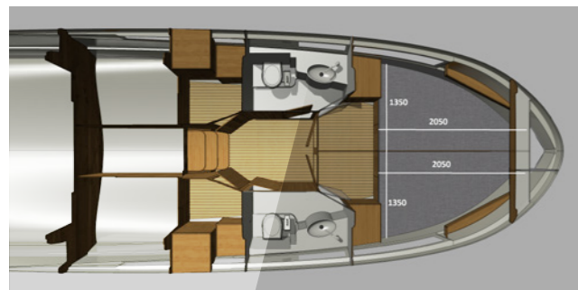
Wersja 2 kabinowa, dwie koje dziobowe / EN / 2-cabin layout, two forward cabins
