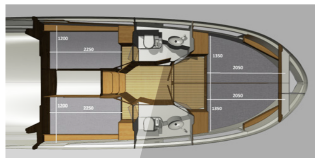
Wersja 4 kabinowa / EN / 4-cabin layout
