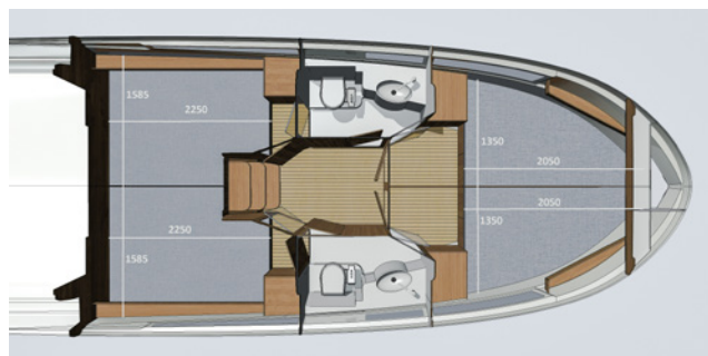
/ EN / 4-cabin layout / DE / 4-Kabinen-Version
