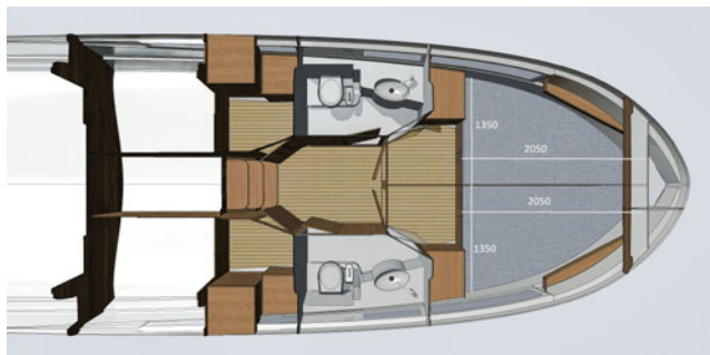
/ EN / 2-cabin layout, two forward cabins / DE / 2-Kabinen-Version, zwei Bugkojen
